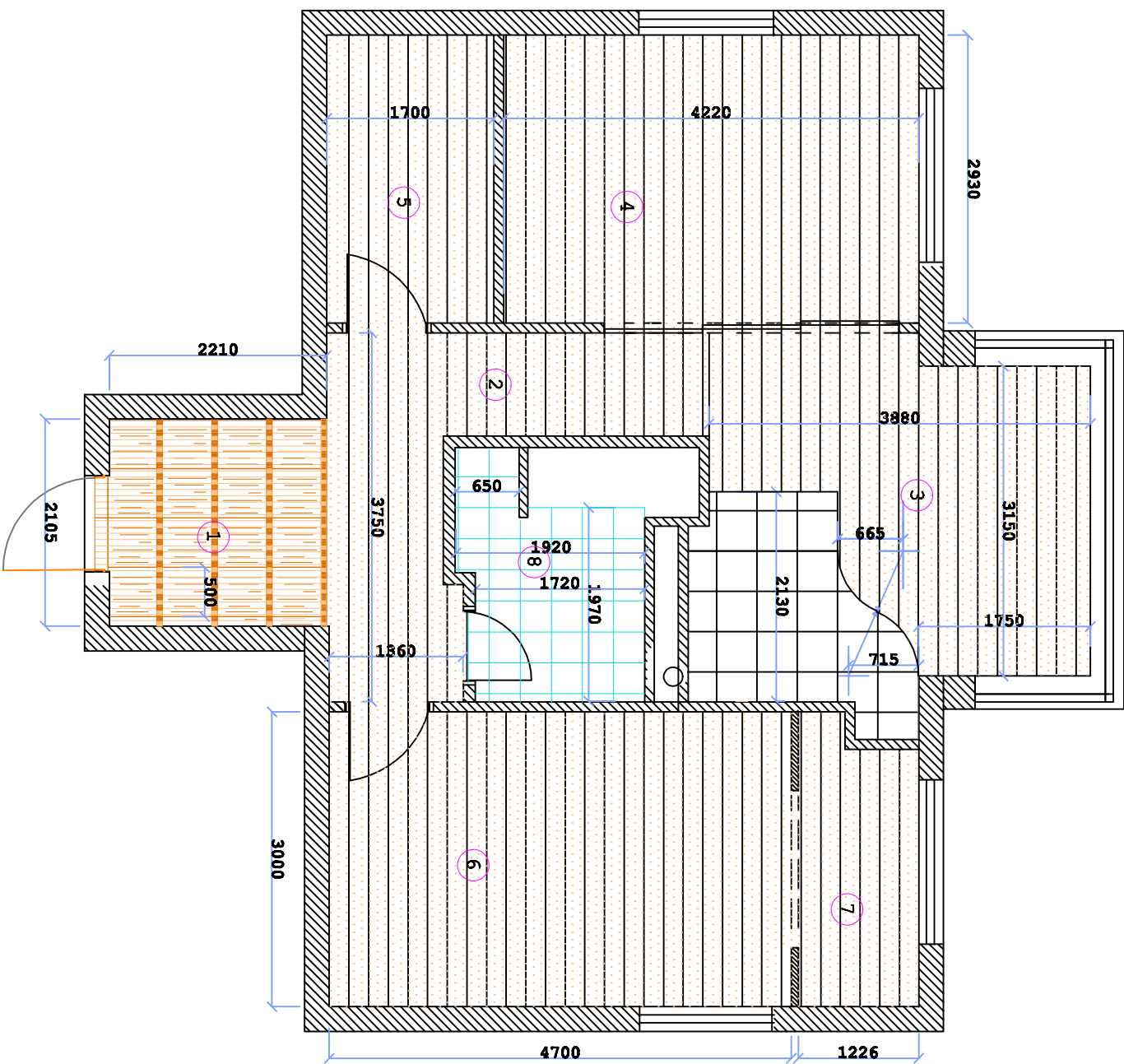
план полов
